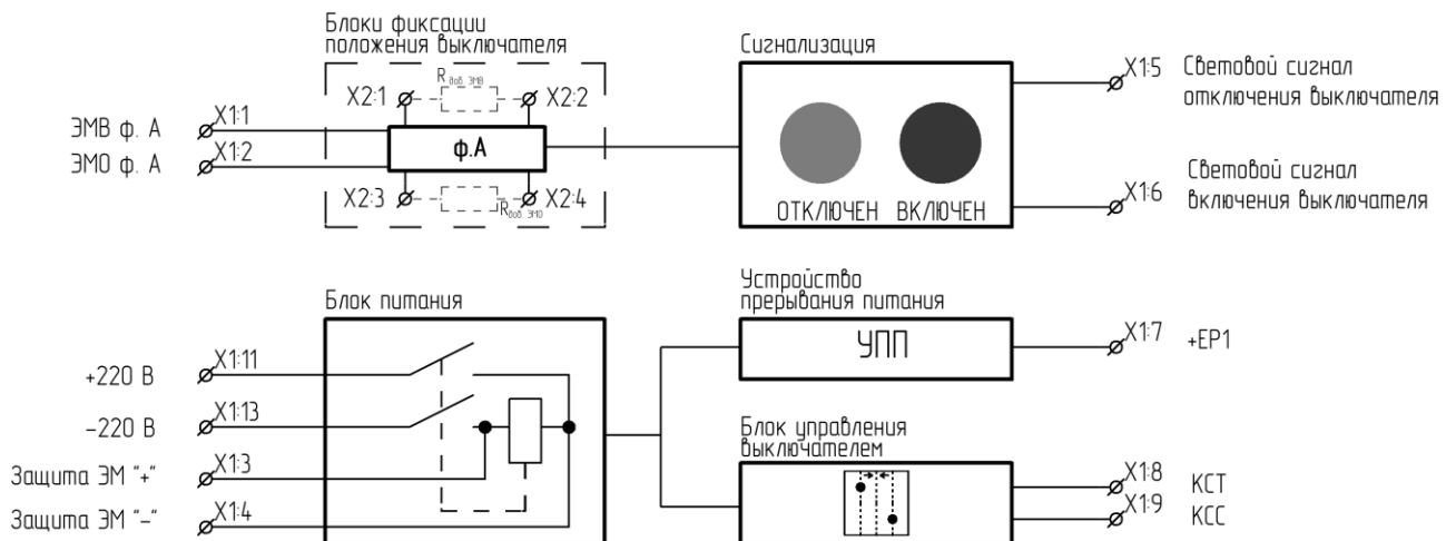
Рисунок 3 – Структурная схема работы модели выключателя с трёхфазным управлением МВ-3
